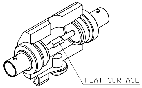
内部構造図
